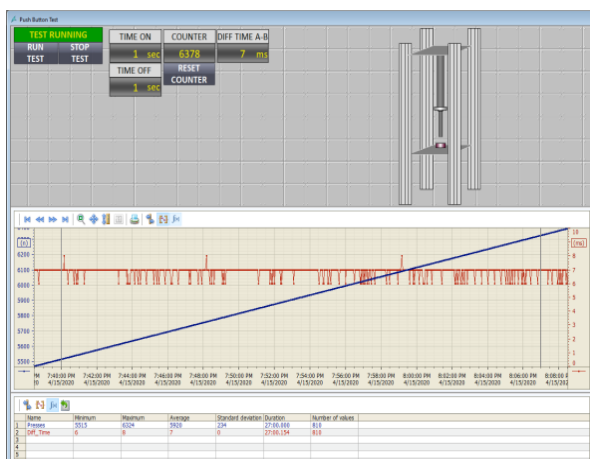
Fig. 9: Scada
