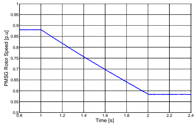
Fig. 7 The PMSG rotor speed
